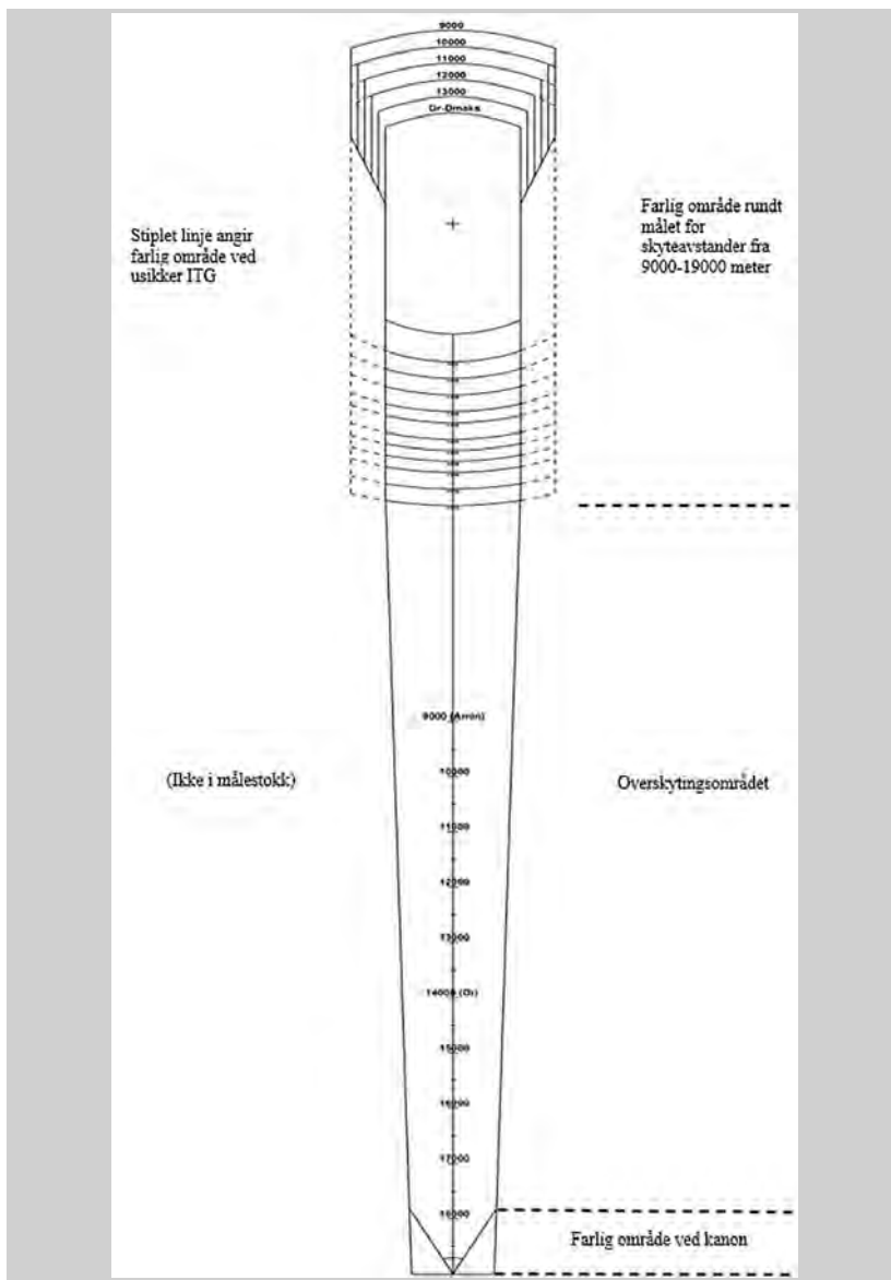
Figur: 3.34 Eksempel på farlig område angitt på sikkerhetsmal
