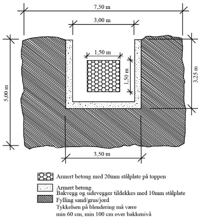
Figur: 3.17 Standplass, sett ovenfra
