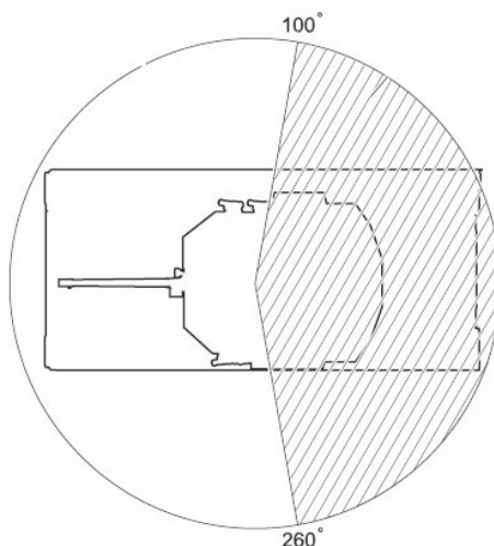
Figur: 3.32 RWS rettebegrensning
