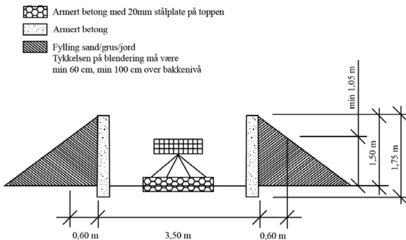
Figur: 3.16 Standplass, sett fra siden
