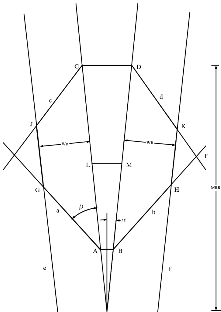
Figur: VI.1 Mal for ammunisjon uten splinter
