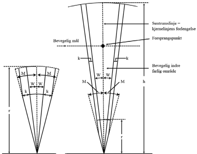
Figur: 3.39 Eksempel på bevægelig indre farlig område ved skyting mot luftmål.
