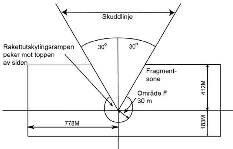
Figur: 2.9 Detaljert skisse av fragmentsonen ved avfyring av eksplosivslange (M58)
